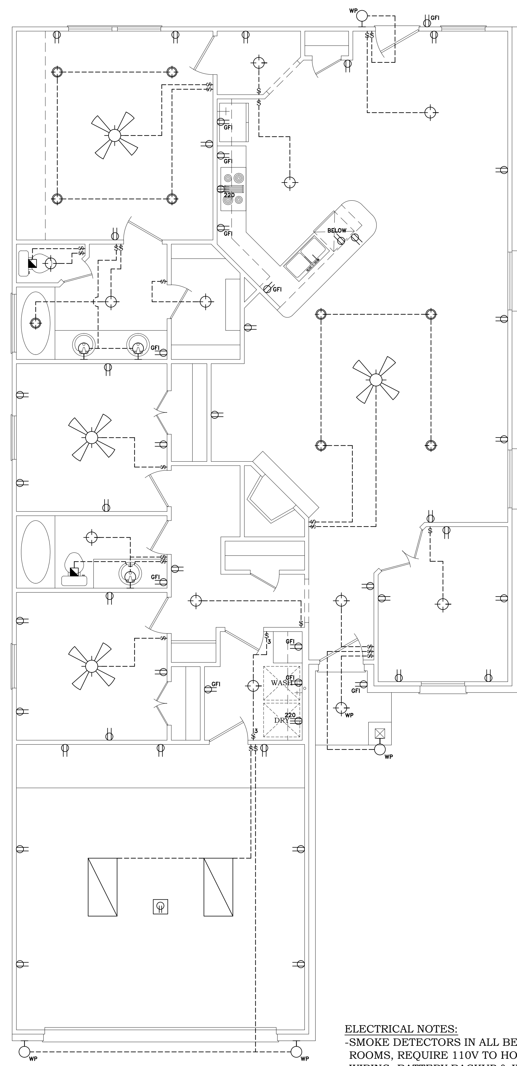
2 ELECTRICAL A2 SCALE: 1/4" = 1'
